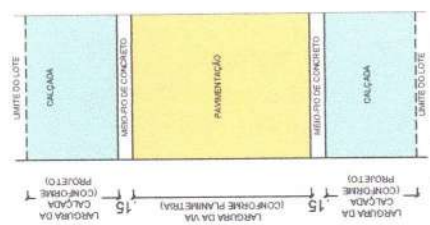
Croqui esquemático - ampliação do planimétrico escala 1:30
